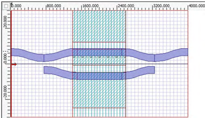
Fig. 1 LN MZM
